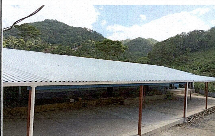
Foto 3: Ampliación de piso y techo con cubierta y estructura tipo pórtico.
