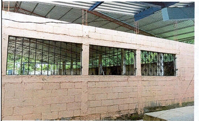
Foto 4: Mejoramiento de ventanales con balcones.
